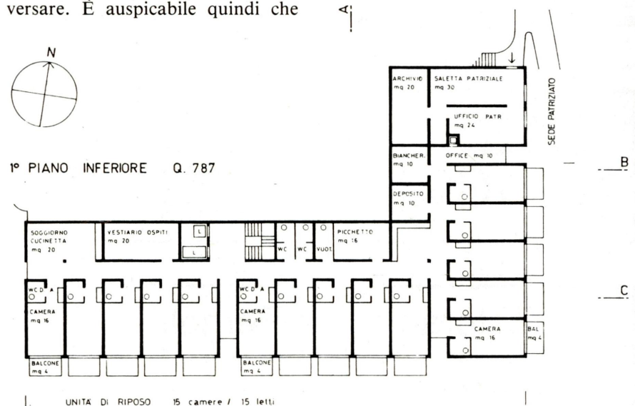
Pianta piano tipo, progetti di massima.
