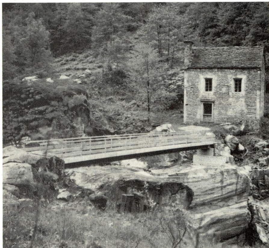
Il ponte ricostruito nell'ambito dei lavori urgenti 1978-1979 per accesso alla sponda destra.
